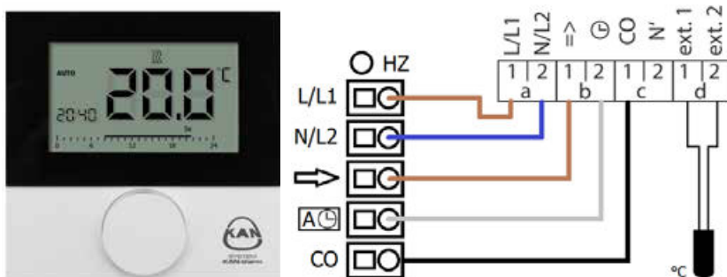
Фиг. 70. Схема на окабеляване на стенен термостат за отопление и охлаждане към клемния блок Basic+ 230V или 24V (с възможност за периодично намаляване на температурата чрез използване на вътрешния му таймер за други стайни термостати)
