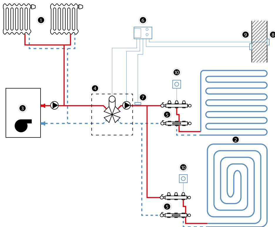
Фиг. 52. Диаграма на централната смесителна система с автоматично регулиране.
