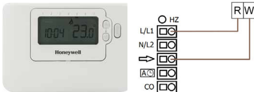
Фиг. 67. Схема на окабеляване на седмичен регулатор към клемен блок Basic+ 230V или 24V (с опция за периодично намаляване на температурата чрез свързване на външен часовник)
