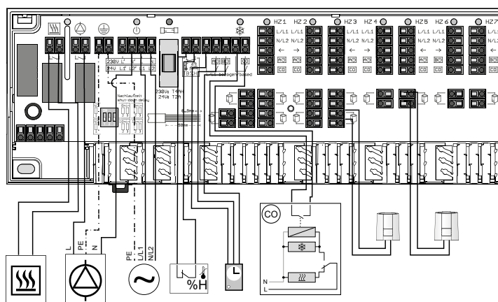
Фиг. 71. Електрически клемен блок Basic+ 230V или 24V. Версията 24V се нуждае от допълнителни 230 - 24 AC към AC преобразувател на мощност
