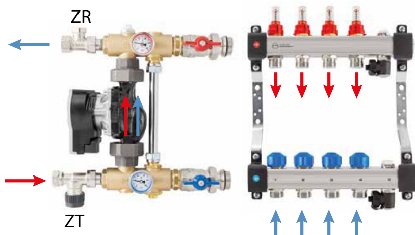
Фиг. 59. Помпена група с константна стойност с UFST разпределител – посоки на потока
