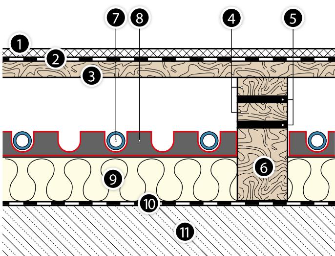
Фиг. 33. Структура на повърхностно еластичен спортен под с подова инсталация изградена от елементите на системата KAN-therm Rail.
