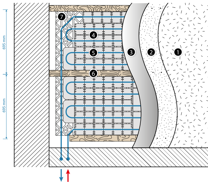
Фиг. 37. Напречно сечение на инсталацията за стеново отопление KAN-therm TBS.
