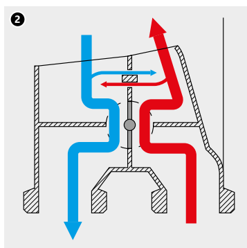
1. Смесител KAN-Bloc с четирипътен вентил и корпус от термоизолация 2. Принцип на работа на четирипътния вентил в смесител KAN-Bloc
