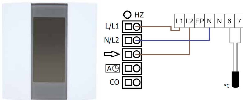
Фиг. 68. Схема на окабеляване на седмичен регулатор за отопление към клемен блок Basic+ 230V (с опция за температурен сензор на пода)
