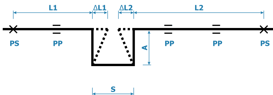
Компенсатор U-образен с фиксирана точка
