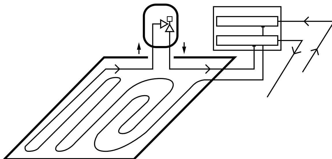
Фиг. 73. Схема на работа– устройството е монтирано на връщащия кръг
