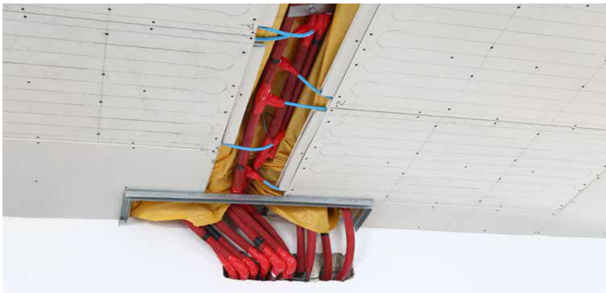
Фиг. 6. Таванна охладителна инсталация с отоплителни и охлаждащи панели на системата KAN-therm Wall.
