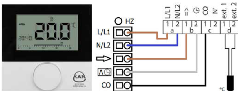
Фиг. 66. Схема на окабеляване на стаен термостат за отопление и охлаждане към клемния блок Basic+ 230V или 24V (с възможност за периодично намаляване на температурата чрез използване на вътрешния му таймер за други стайни термостати)
